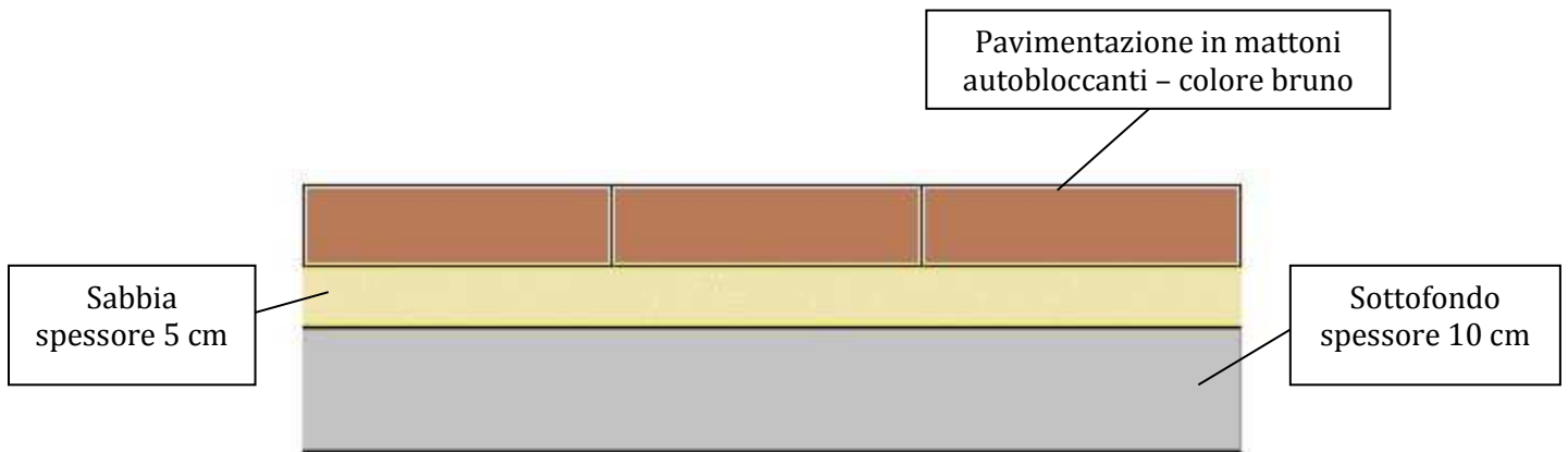
Elaborato grafico - Sezione nuova pavimentazione
